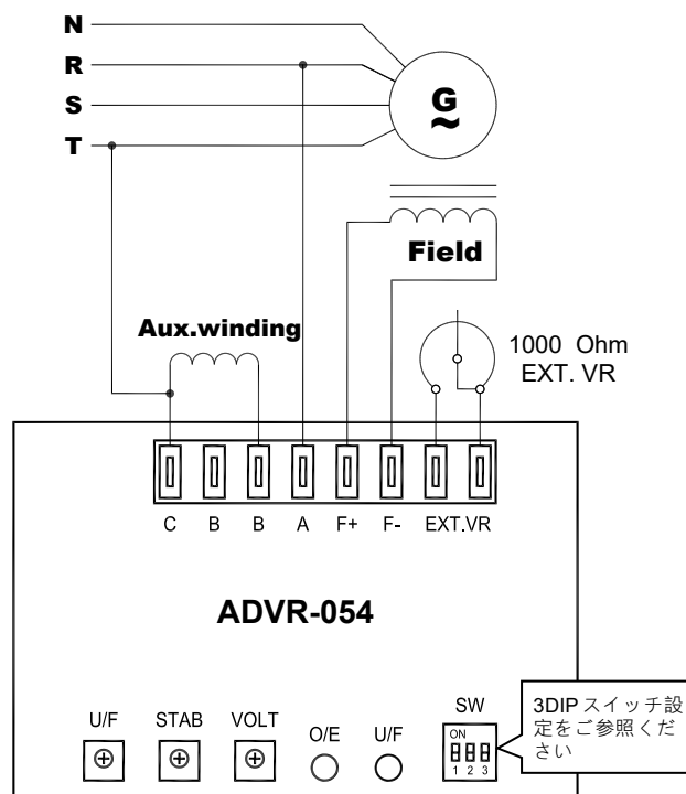
図 6 補助巻線
