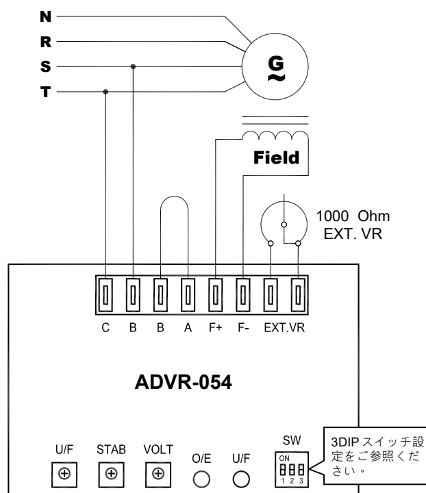
図 4 検出電圧入力 170 – 260V (方法 2)
