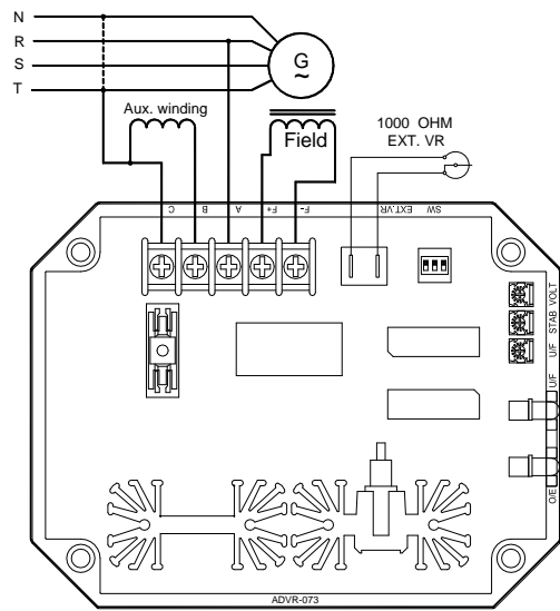
圖七 輔助繞組接線
