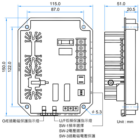
圖二 尺寸圖
