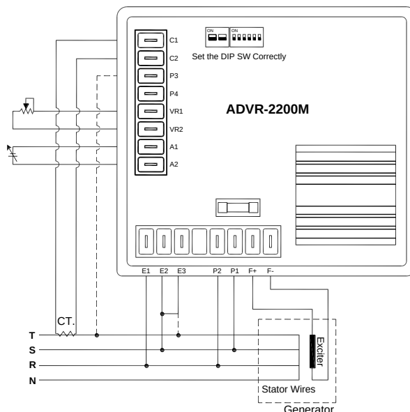
圖四 自勵式接線圖
