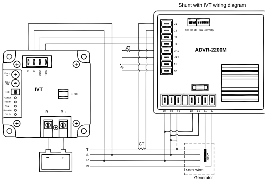
圖六 ADVR-2200M & IVT-1260 / IVT-2460 接線圖
