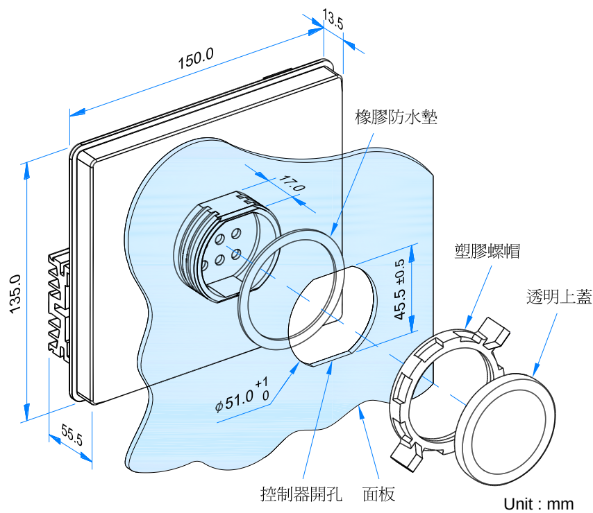
圖一 尺寸圖
