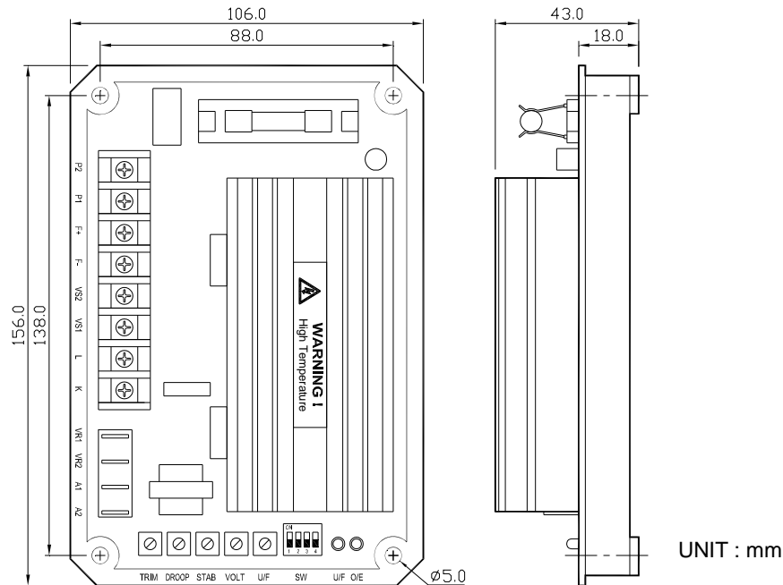
圖一 尺寸圖
