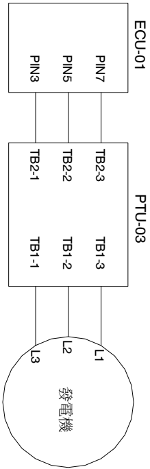
發電機電壓208~240VAC接線方式 PS : 功能設定選項38 設定為 "0"
